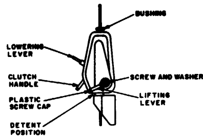
F. GRIPHOIST
